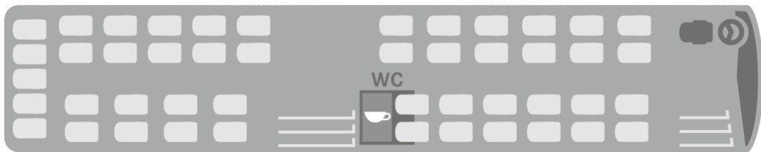
Variante 1 S 416 UL - 47 sedili + WC + cucina di bordo
