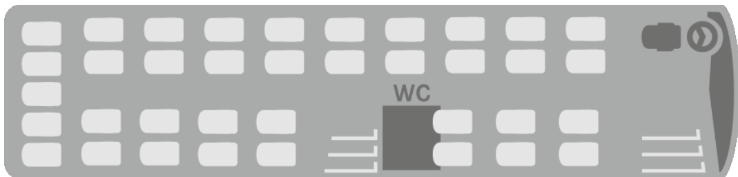
Variante 1 S 412 UL - 37 sièges + WC
