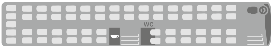
Variante 2 S 519 HD - 4 estrellas - 59 asientos + aseo + cocina de a bordo
