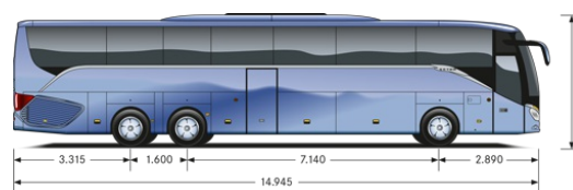
Todas las medidas se indican en milímetros.
