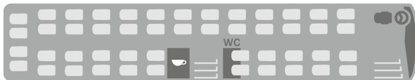
Varianta 2 S 516 HD - 4 Stele - 48 locuri - clasa 3 + WC + bucătărie
