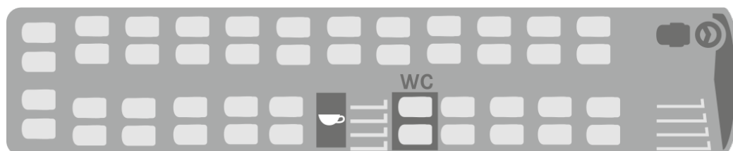
Varianta 2 S 515 HDH - 4 Stele - 46 locuri + WC + bucătărie
