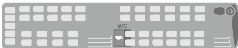
Wariant 1 S 416 UL - 47 siedzeń + WC + kuchnia pokładowa
