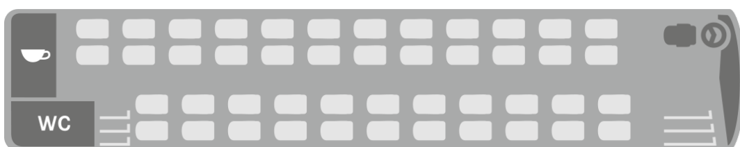
Varianta 2 S 516 MD - 4 Stele - 46 locuri + WC + bucătărie
