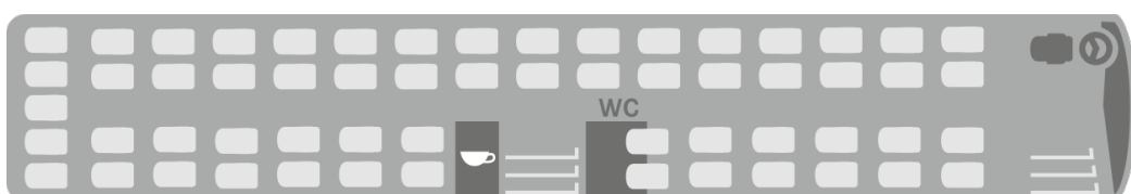
Variant 2 S 519 HD - 4 sterren - 59 stoelen + toilet + boardkeuken
