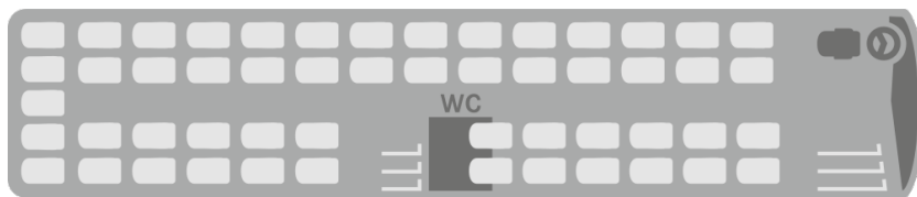
Έκδοση μοντέλου 1 S 516 HD - 3 αστέρια - 53 θέσεις καθήμενων + WC
