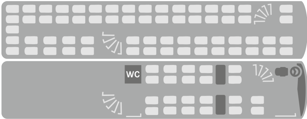
Variante 1: S 431 DT - 3 Sterne - 85 Sitzplätze + WC
