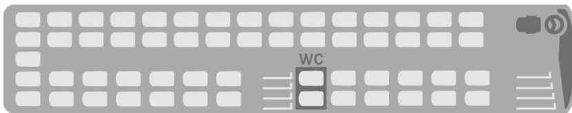
Variante 1: S 516 HDH - 3 Sterne - 57 Sitzplätze + WC
